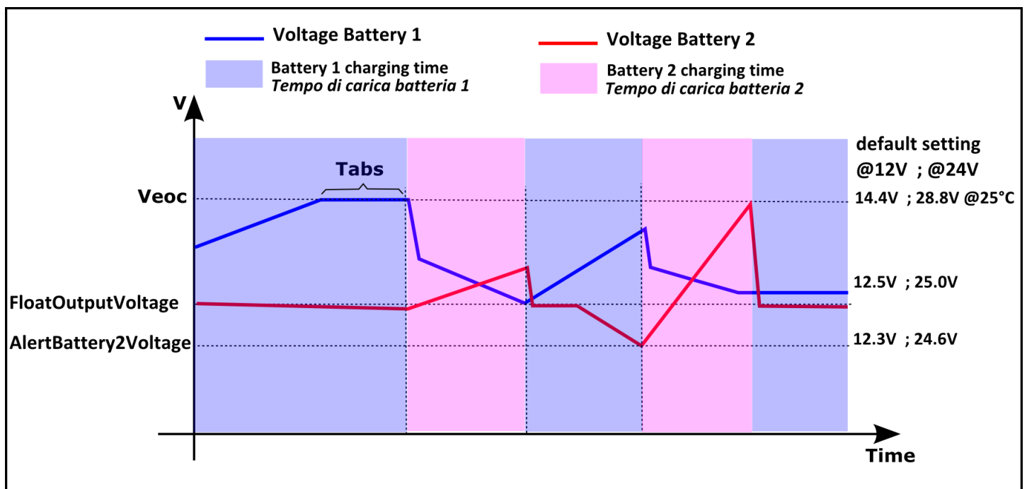
Fig. 3 Gestione batteria 1 e batteria 2
