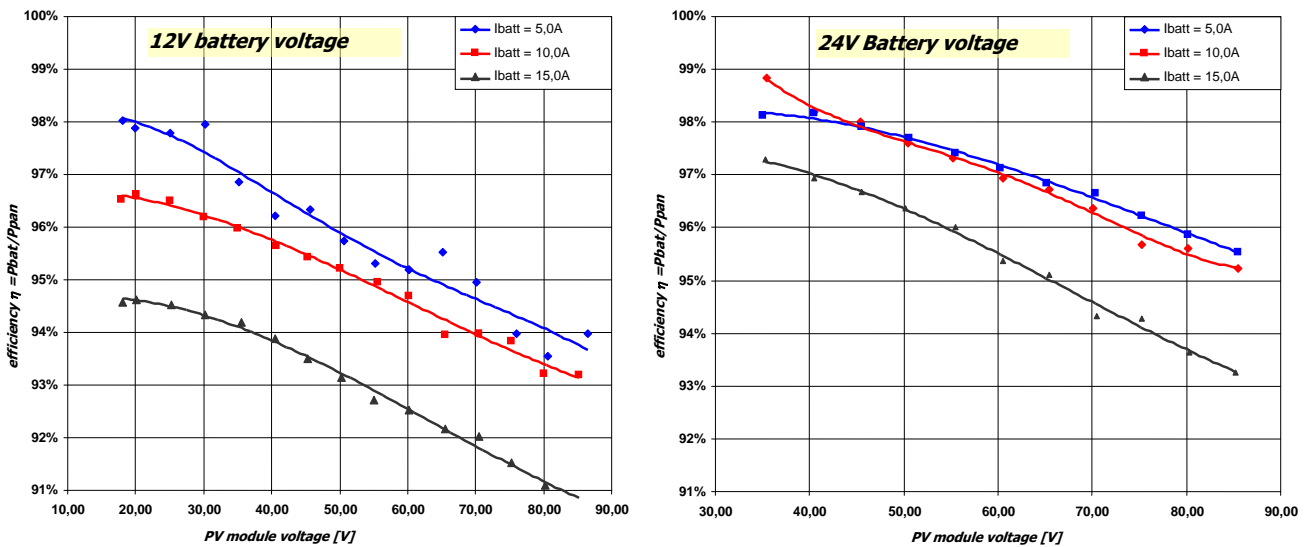
Fig. 7 Rendement du dispositif WRM15 - dualB en fonction de la tension du panneau pour un système à 12V et 24V
