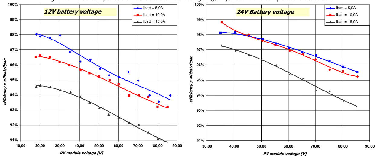
Fig. 7 Rendimiento del WRM15 - dualB en función de la tensión de panel para sistema de 12 V y 24 V
