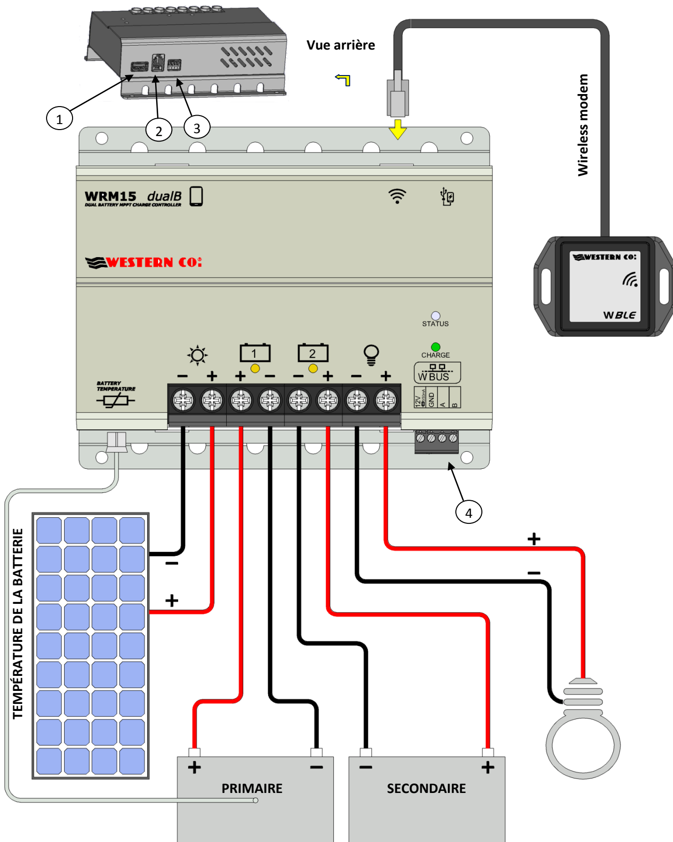
Fig. 2 Schéma de branchement
