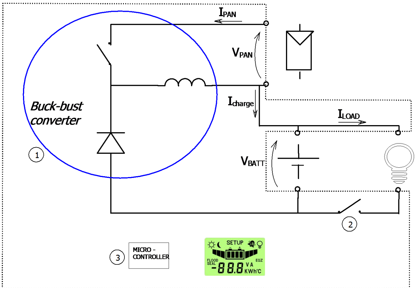
Abb. 1 Prinzipschema
