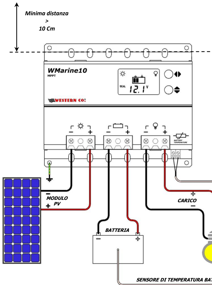
Fig. 2 Schema di collegamento
