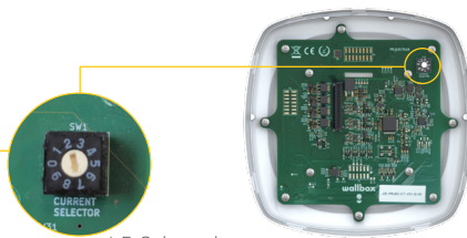
I-5: Seletor de corrente
