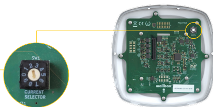
I-5 : Sélecteur d'intensité
