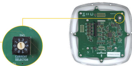
I-5: Selettore di corrente
