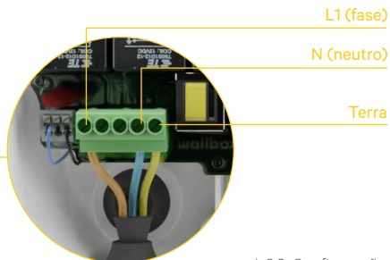
I-6.2: Configuração monofásica (1P)
