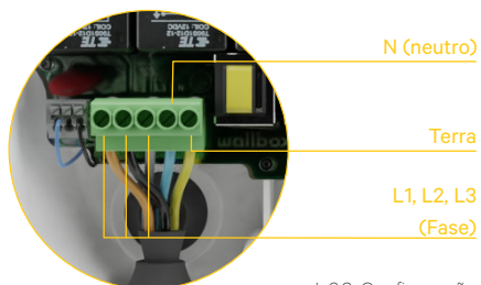
I-6.3: Configuração trifásica (3P)
