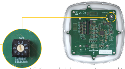
I-5: Keuzeschakelaar voor stroomsterkte
