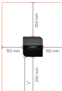
I-1: Monteringsområde
