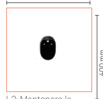
I-2: Mantenere la distanza intorno al supporto per connettore di ricarica
