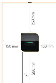
I-1: Monteringsyta
