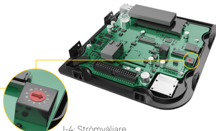
I-4: Strömväljare
