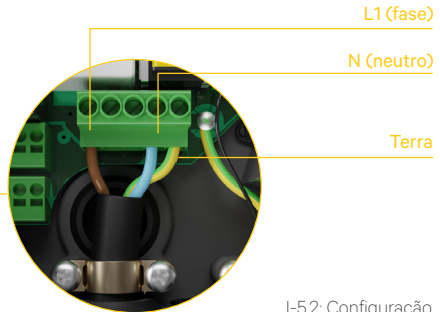
I-5.2: Configuração monofásica (1P)
