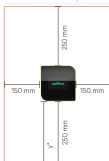
I-1: Área de instalação
