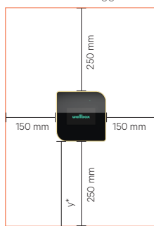
I-1: Area di montaggio
