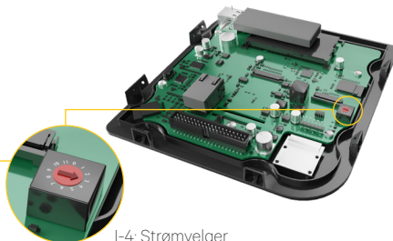
I-4: Strømvelger
