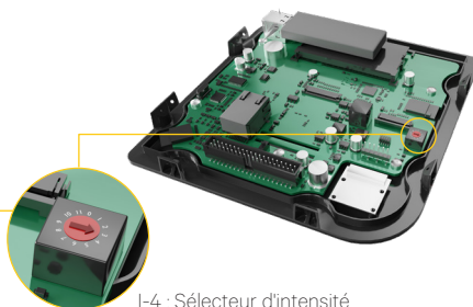
I-4 : Sélecteur d'intensité
